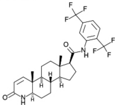
Dutasterid
